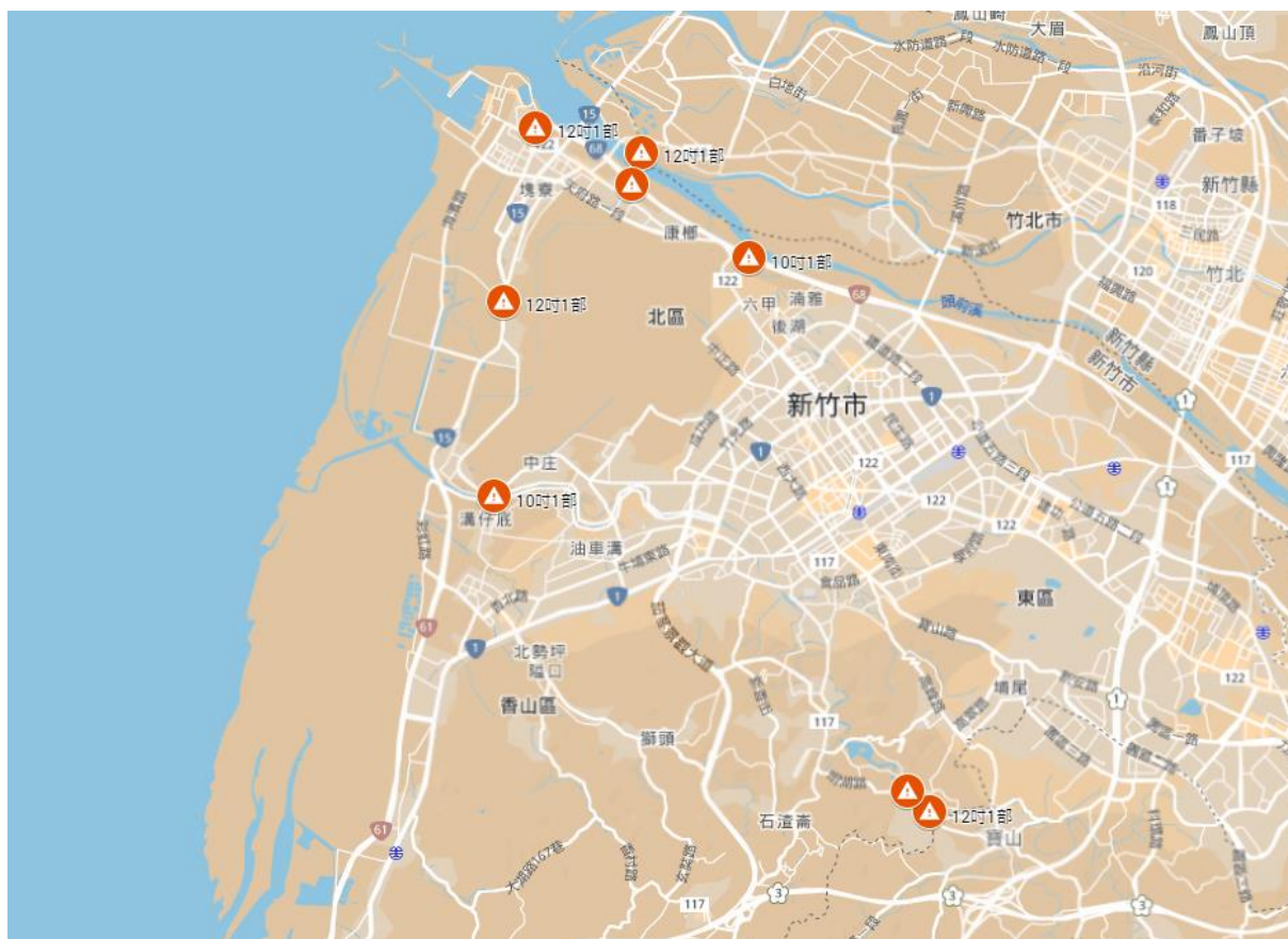
圖 3-6、移動式抽水機預佈位置圖
